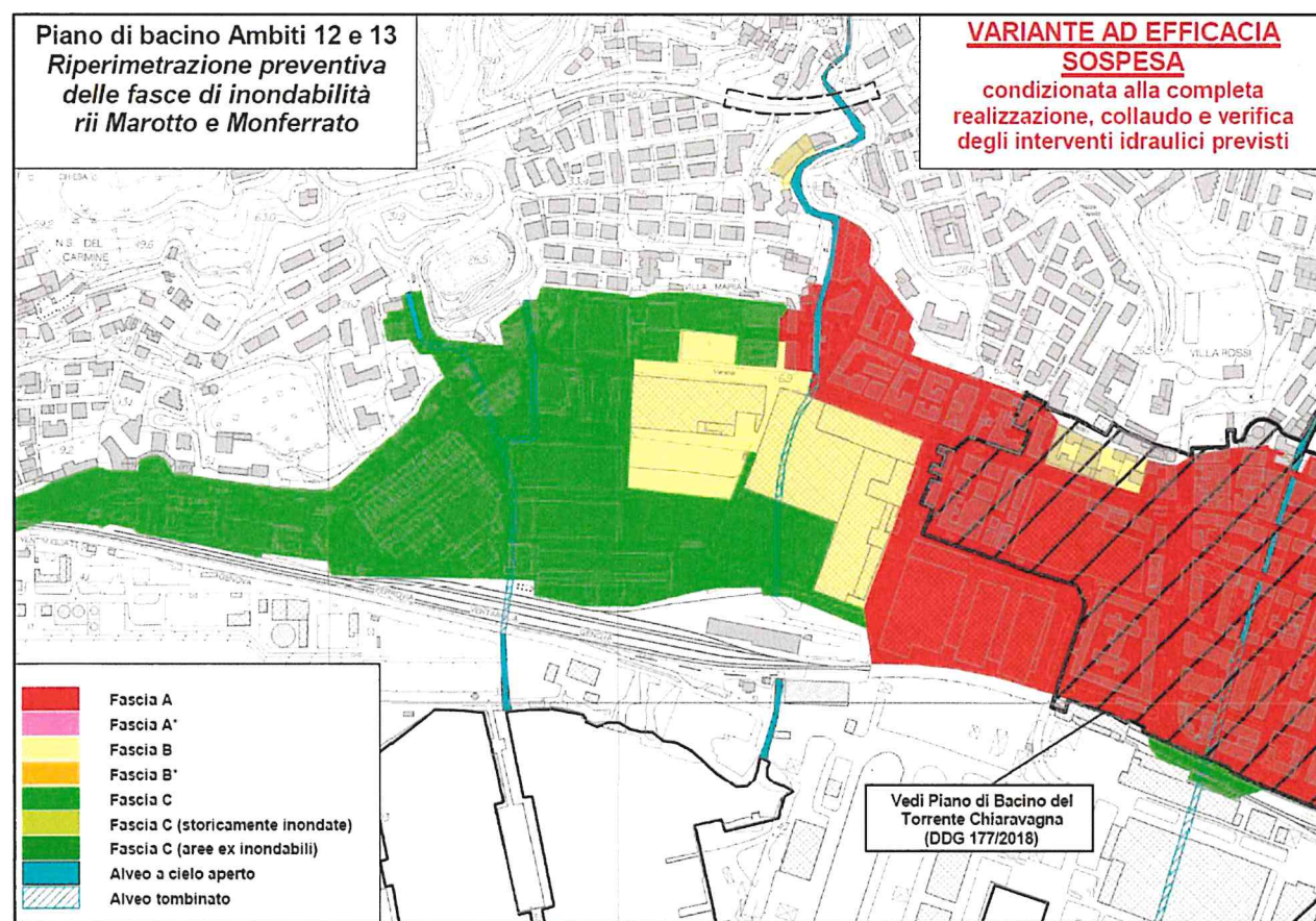
Carta delle fasce di inondabilità – riperimetrazione ad efficacia sospesa
