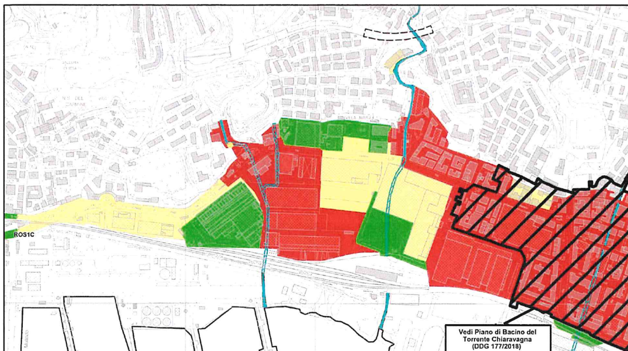
Carta delle fasce di inondabilità – piano vigente
