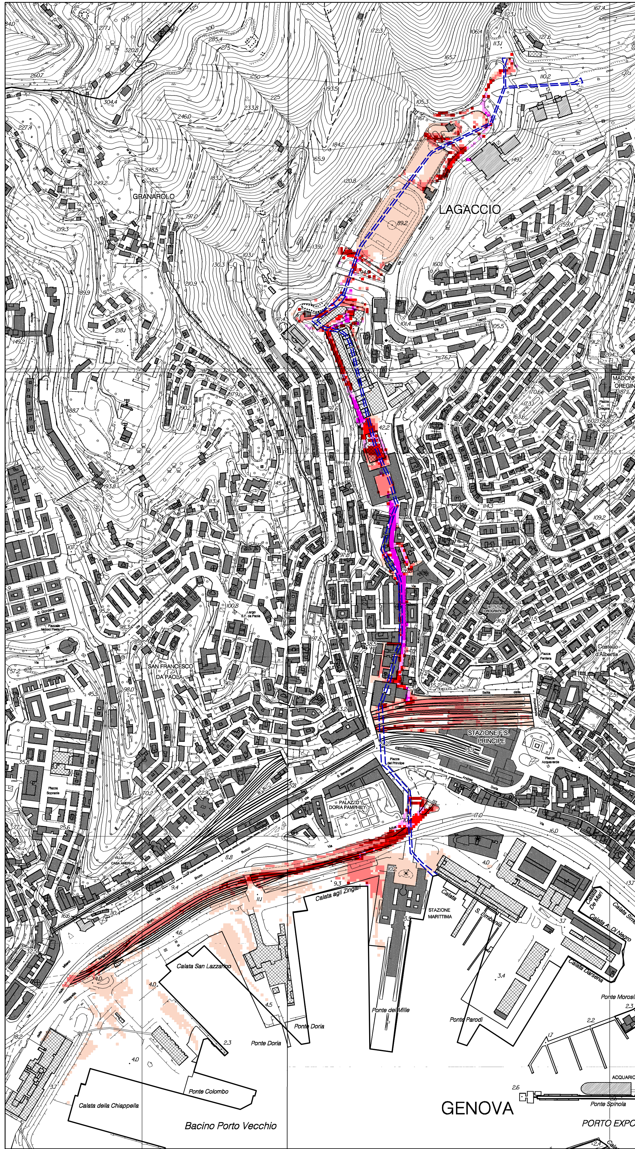
Per tempo di ritorno Tr = 500 anni
