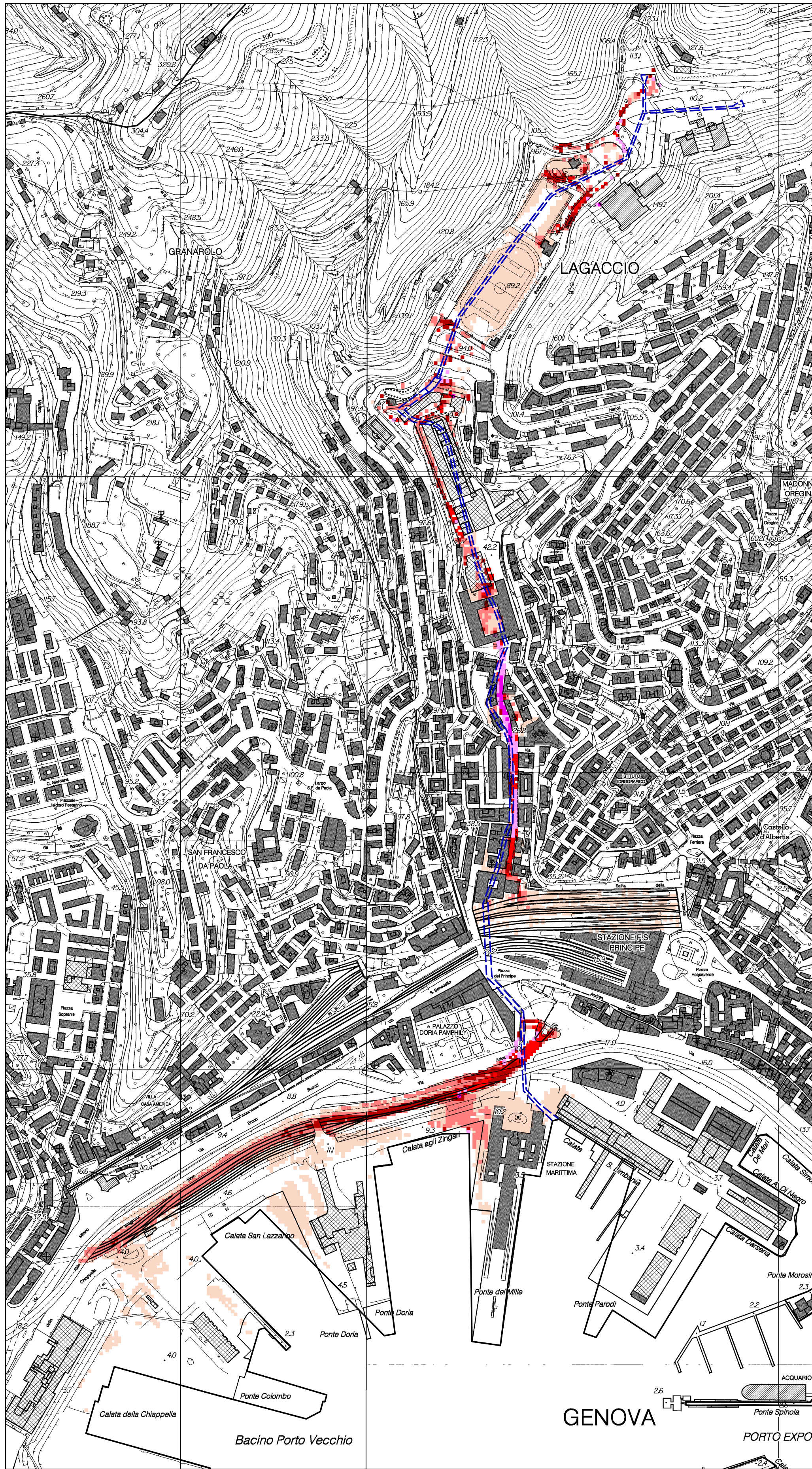
Per tempo di ritorno Tr = 50 anni
