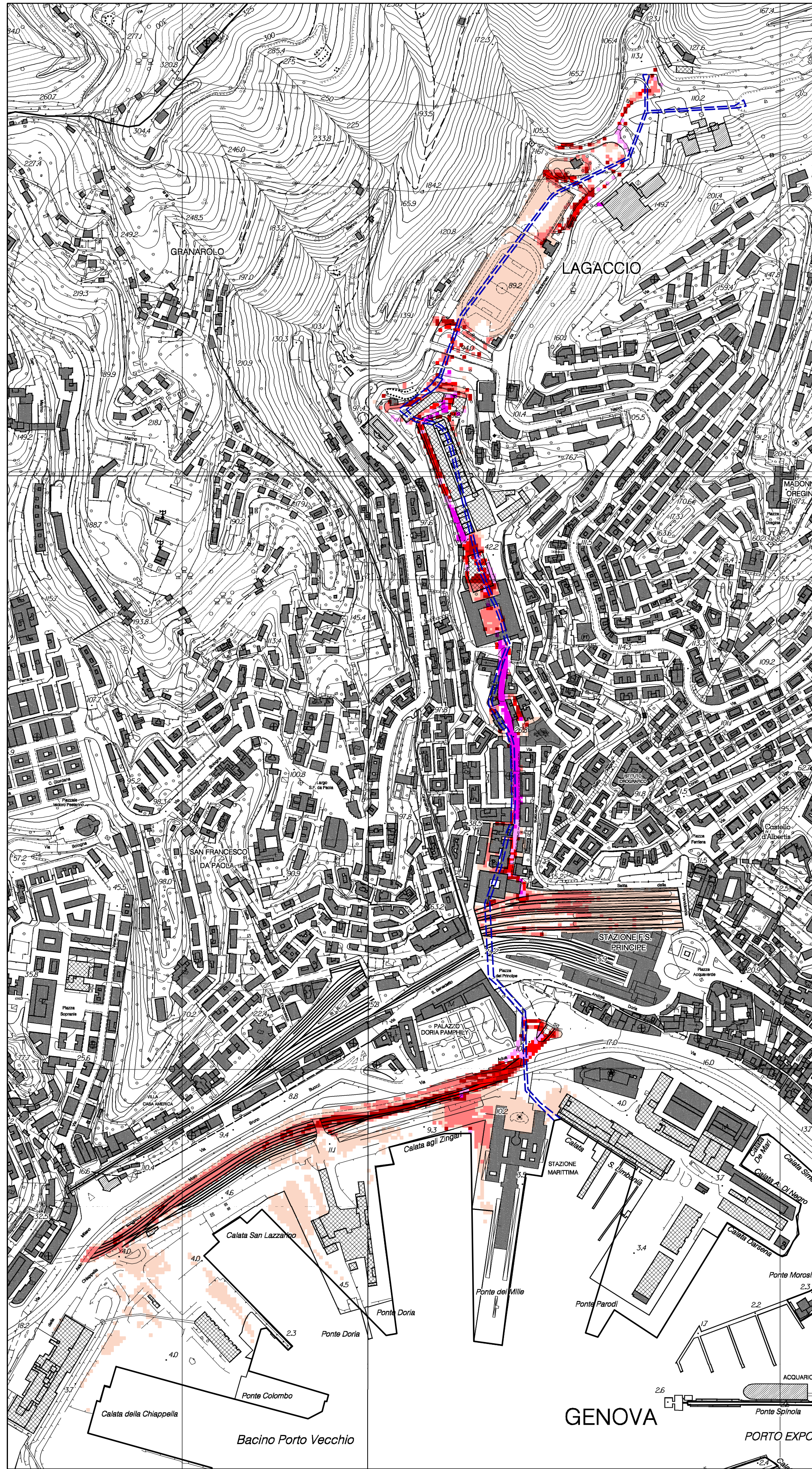
Per tempo di ritorno Tr = 200 anni
