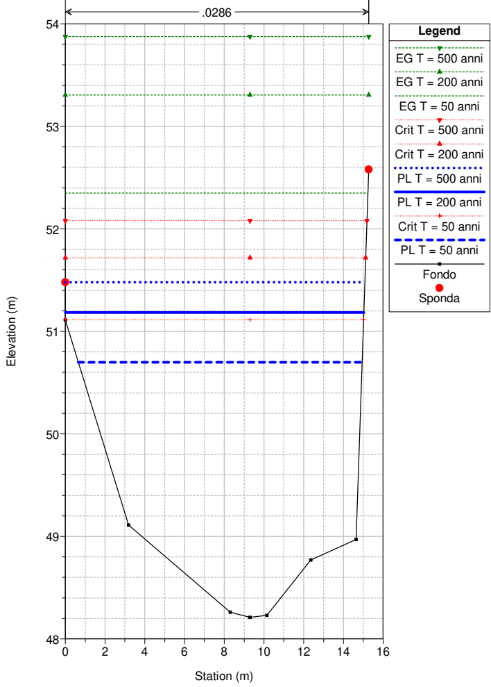
Variante_SBiagio Plan: STATO ATTUALE_ks35 River = Torrente Reach = VERBONE RS = 20 Sezione 2
