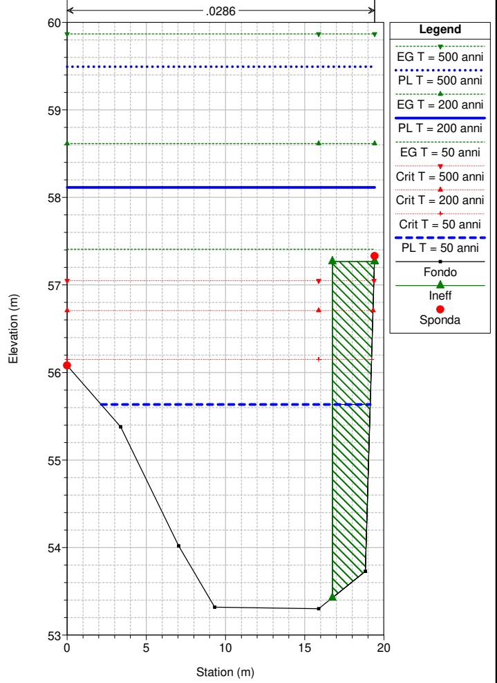
Variante_SBiagio Plan: STATO ATTUALE_ks35 River = Torrente Reach = VERBONE RS = 251 Sezione 25.1 imm.te monte ponte
