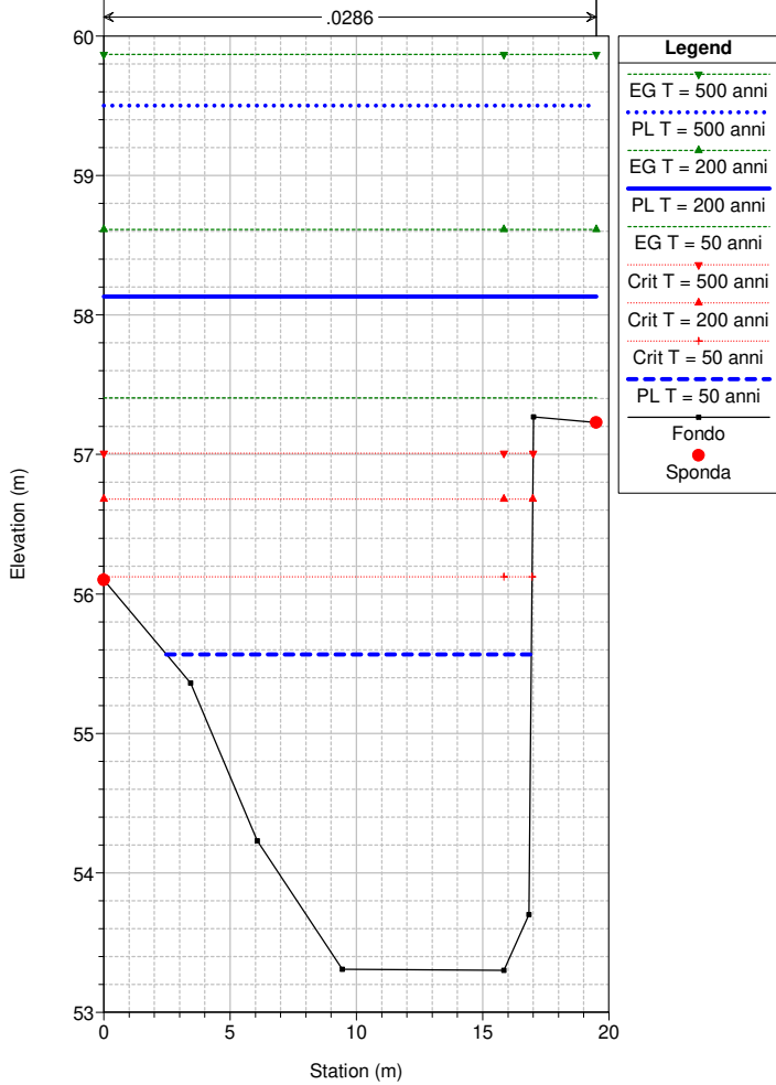
Variante_SBiagio Plan: STATO ATTUALE_ks35 River = Torrente Reach = VERBONE RS = 260 Sezione 26
