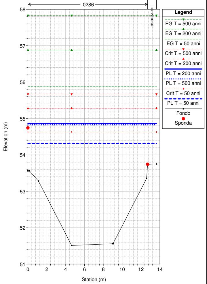
Variante_SBiagio Plan: STATO ATTUALE_ks35 River = Torrente Reach = VERBONE RS = 165 Sezione 16 bis
