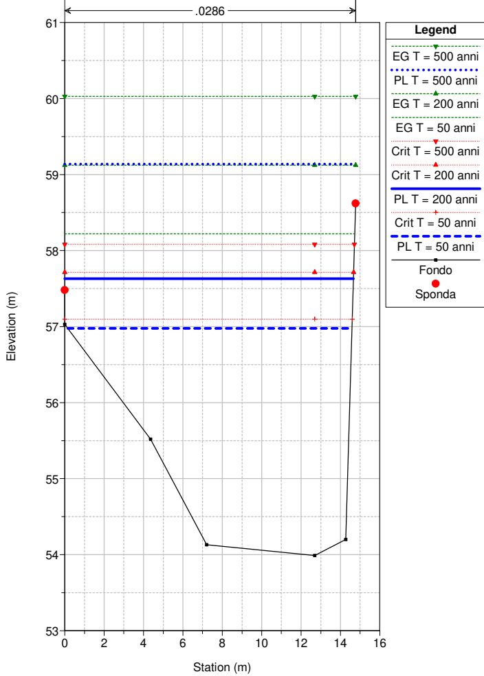
Variante_SBiagio Plan: STATO ATTUALE_ks35 River = Torrente Reach = VERBONE RS = 300 Sezione 30
