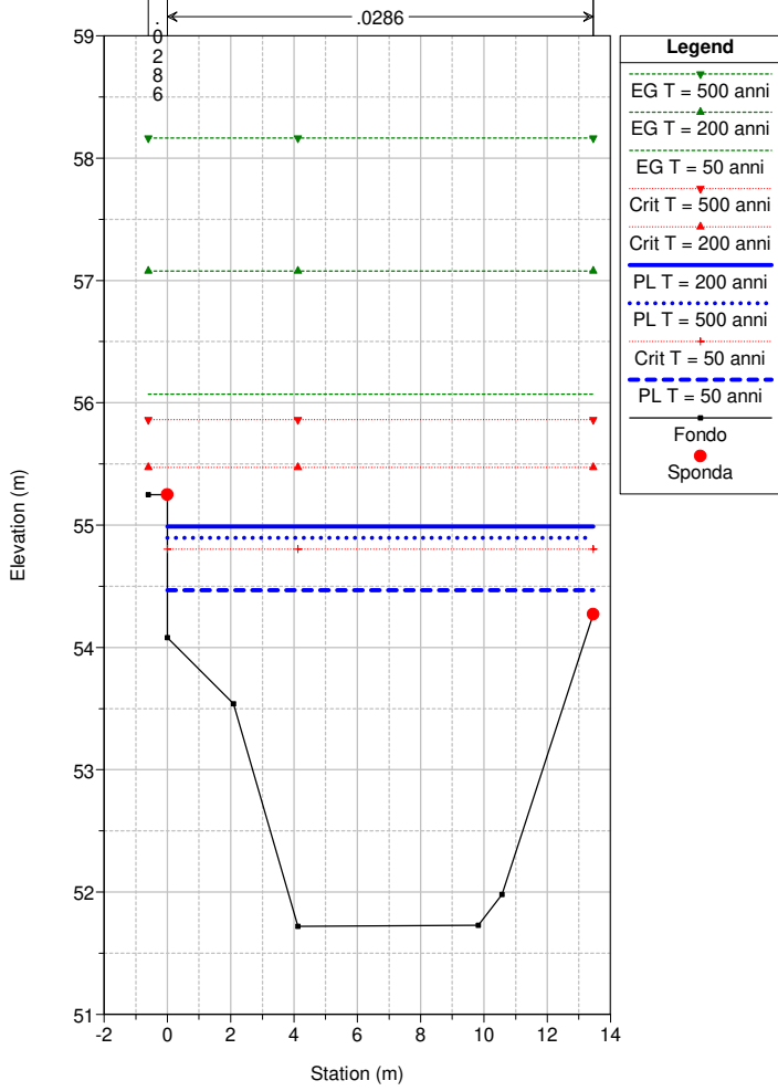
Variante_SBiagio Plan: STATO ATTUALE_ks35 River = Torrente Reach = VERBONE RS = 170 Sezione 17
