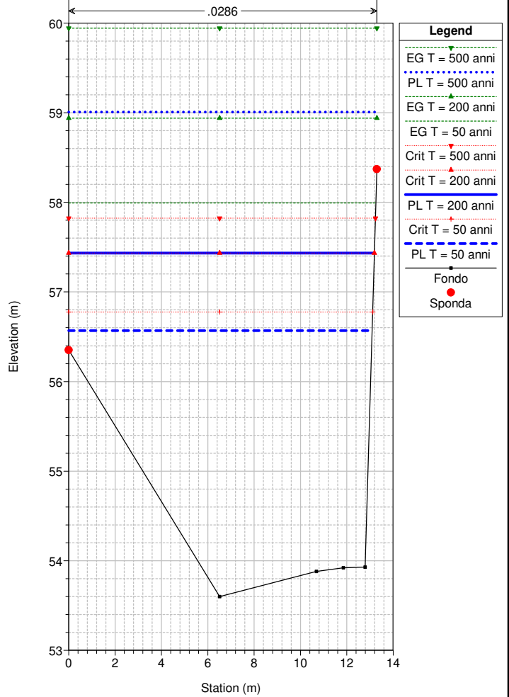
Variante_SBiagio Plan: STATO ATTUALE_ks35 River = Torrente Reach = VERBONE RS = 290 Sezione 29
