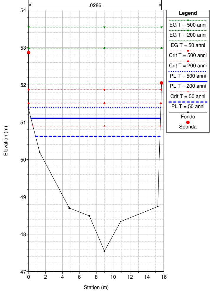
Variante_SBiagio Plan: STATO ATTUALE_ks35 River = Torrente Reach = VERBONE RS = 10 Sezione 1
