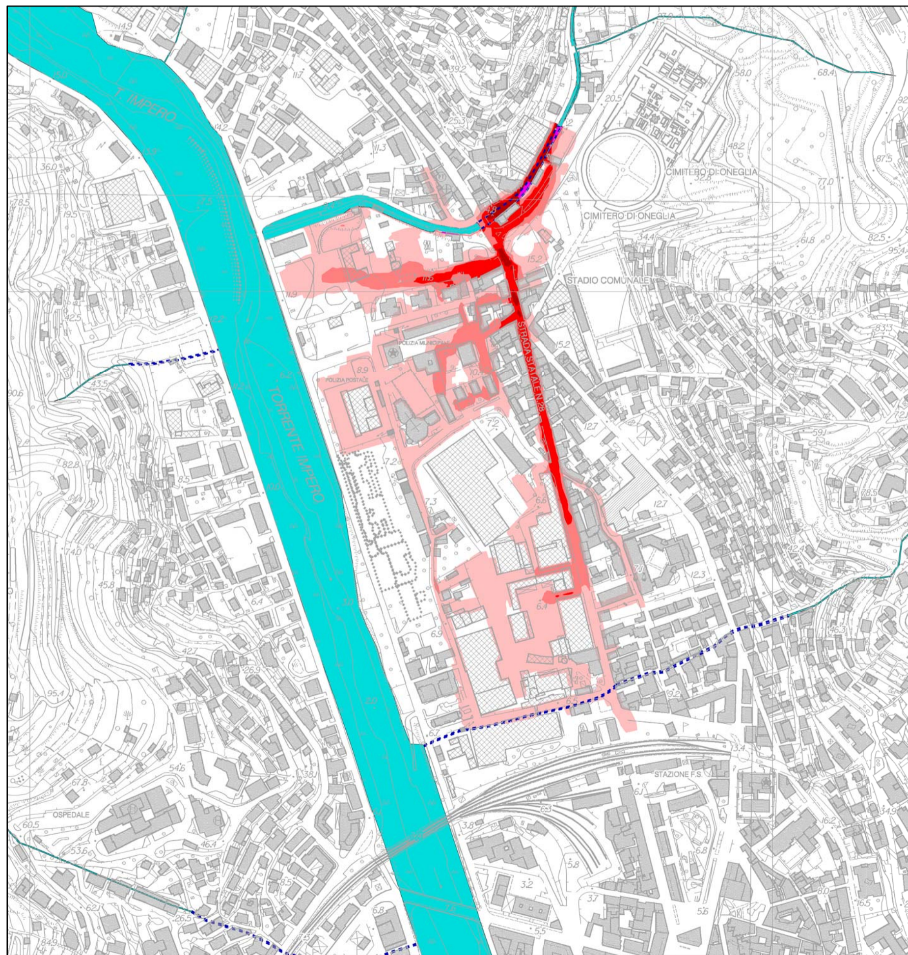
Velocità di scorrimento per Tr = 200 anni
