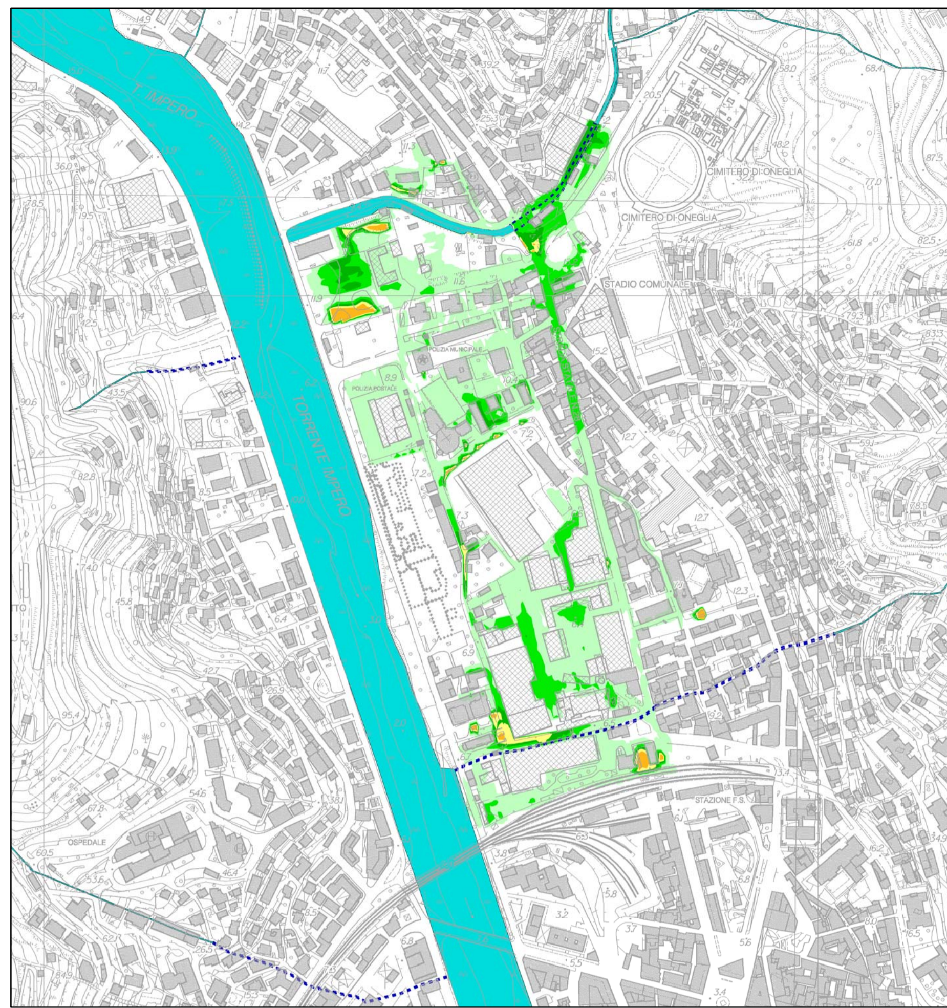
Tiranti idrici massimi per Tr = 500 anni
