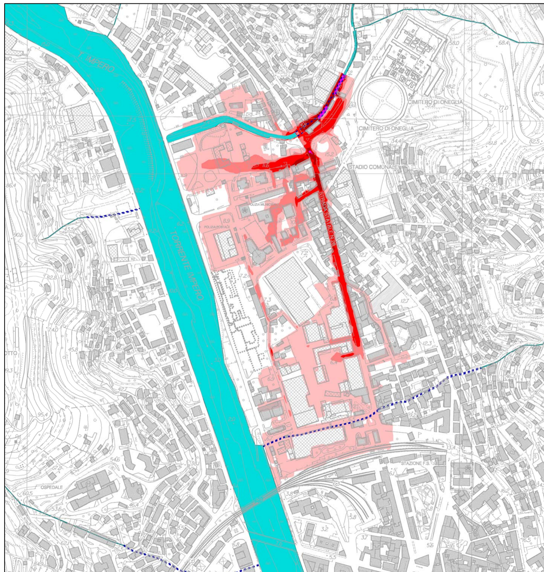
Velocità di scorrimento per Tr = 500 anni
