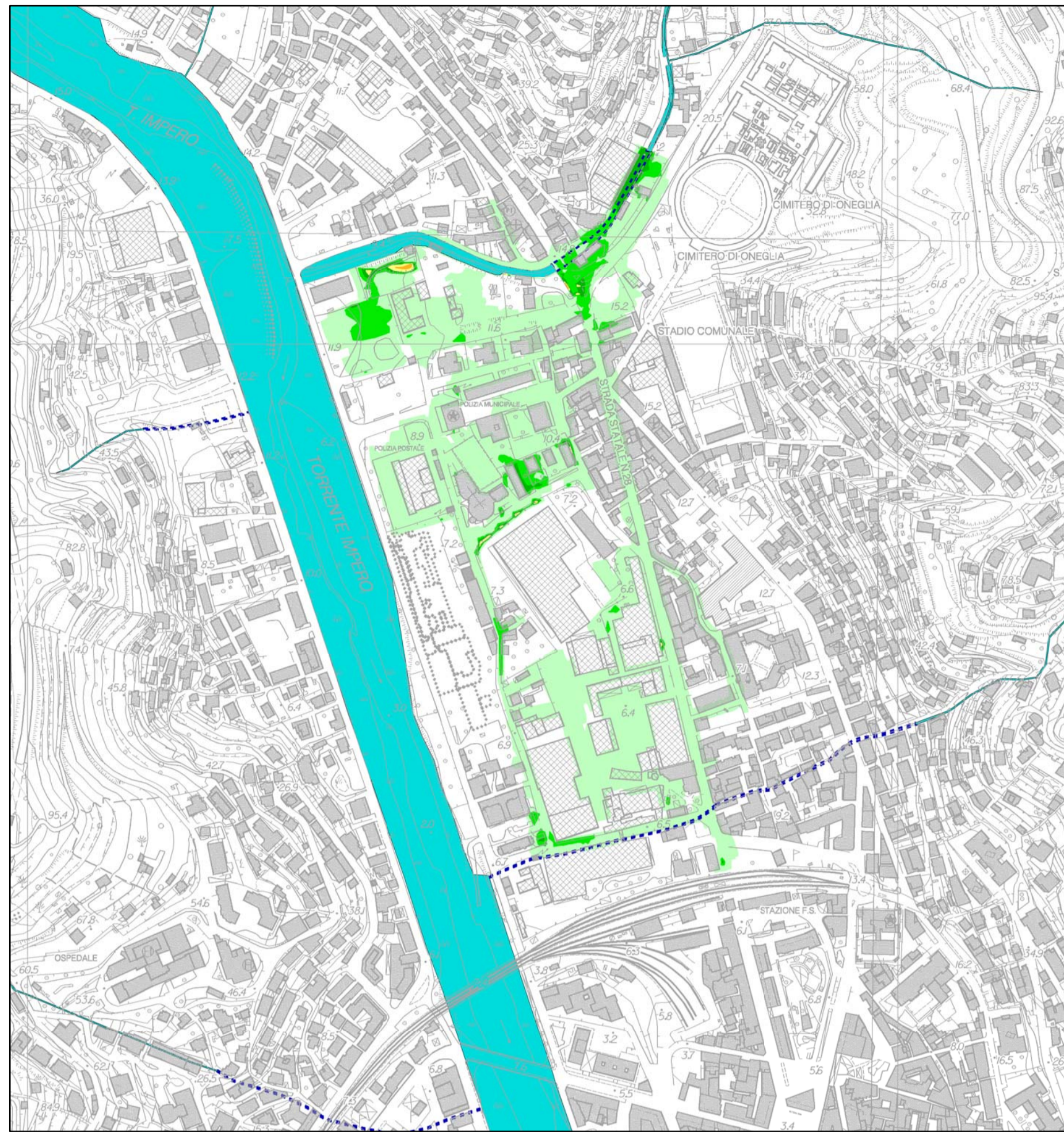
Tiranti idrici massimi per Tr = 200 anni
