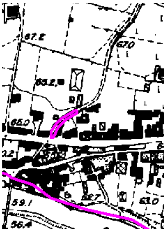
Figura 3.5.3.2.4 – Area Storicamente inondata per il Rio Marassano
