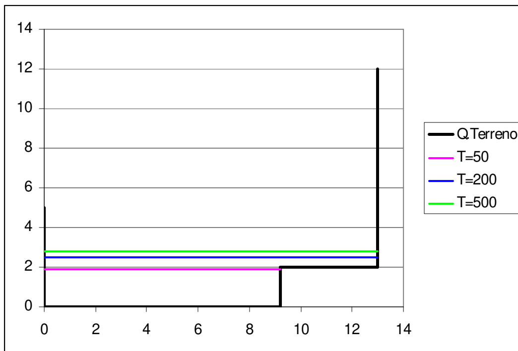
Figura 3.5.3.1.3 – Livelli di piena per il Rio Gallinaro. La portata duecentennale determina l'allagamento della strada sterrata.
